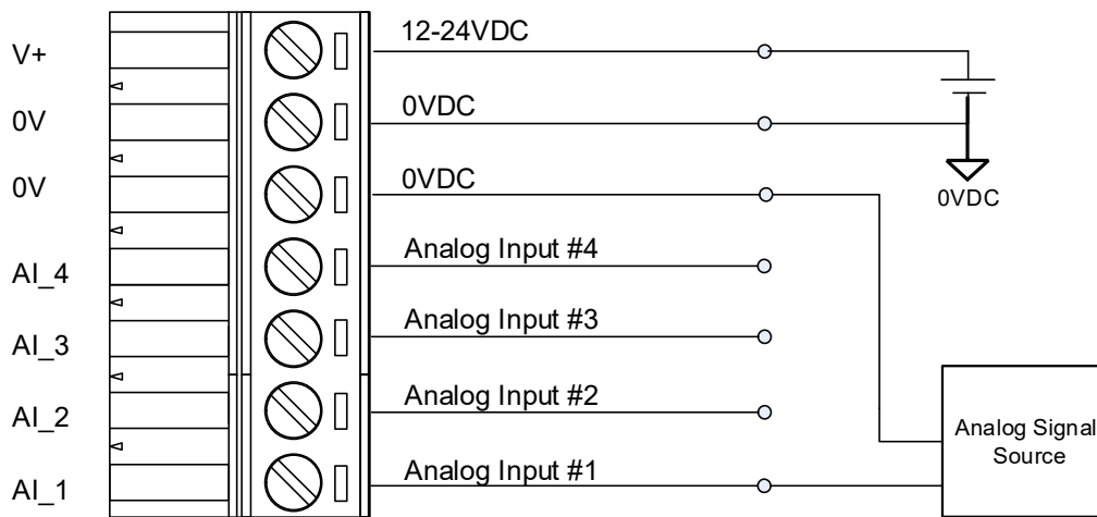
Analog Input
